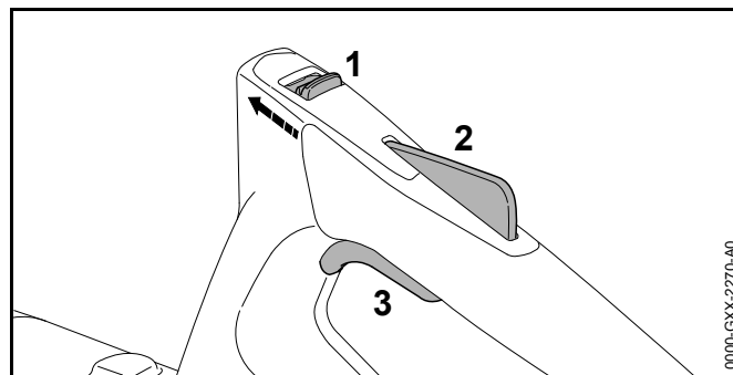
Verrou de retenue (1), bouton de blocage de la gâchette (2) et gâchette (3)
